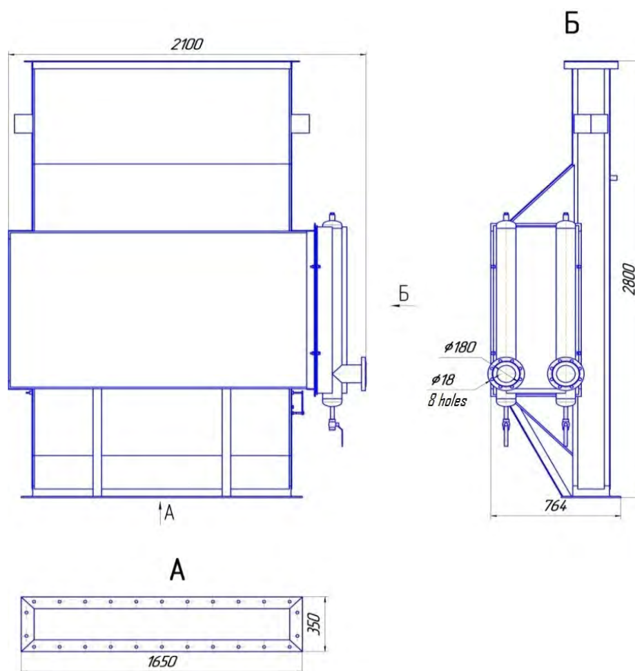
Габаритный чертеж утилизатора тепла для ПТБ
