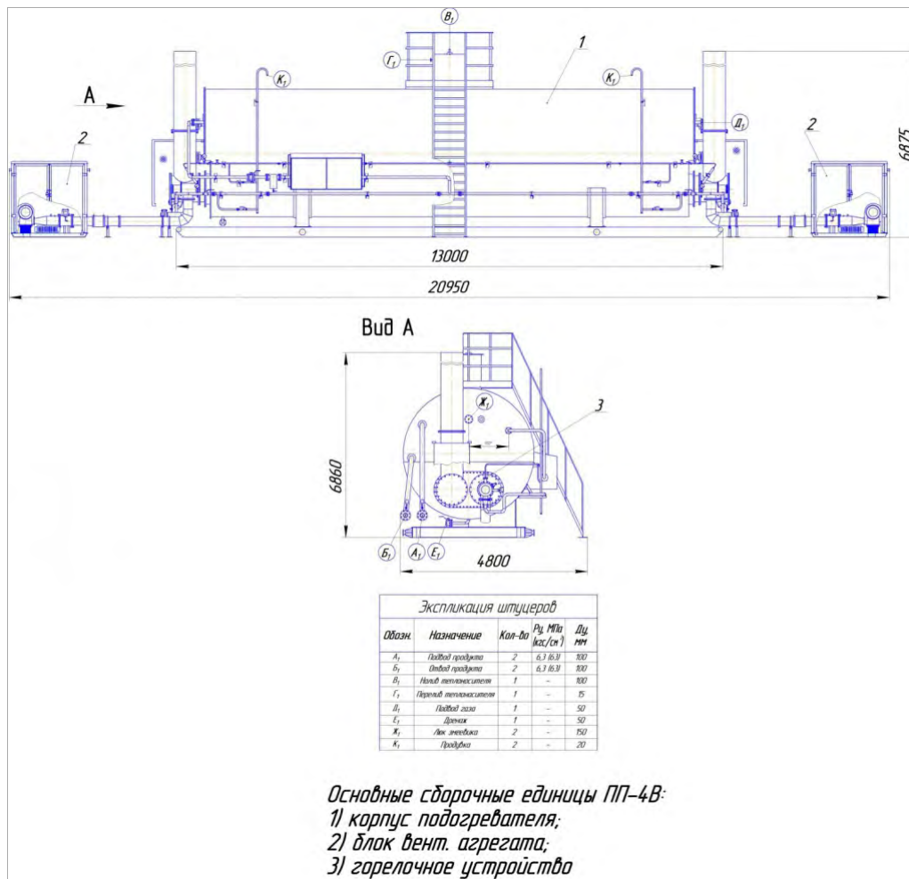
Габаритный чертеж ПП-4В.
